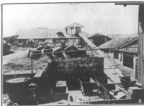
Vista parcial de la planta de fabricar ladrillos en la Alfarería del señor Salvador Garriga.
