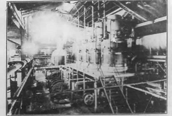
Un aspecto interior de la casa de calderas en el Central "Portugalete".
