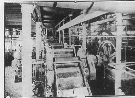
Vista de los trapiches del Central "Portugalete", en Palmira.
