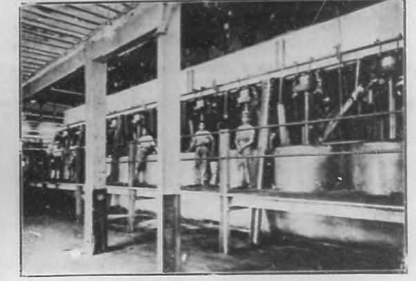
Departamento de centrífugas del Central "Portugalete".
