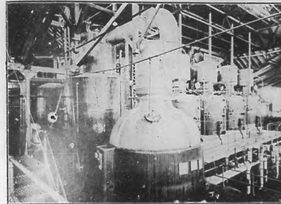
Tachos de vacío y cuádruple-efecto del Central "Portugalete".
