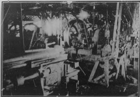
Vista parcial del taller de maquinarias de la Alfarería del Sr. Salvador Garriga.
